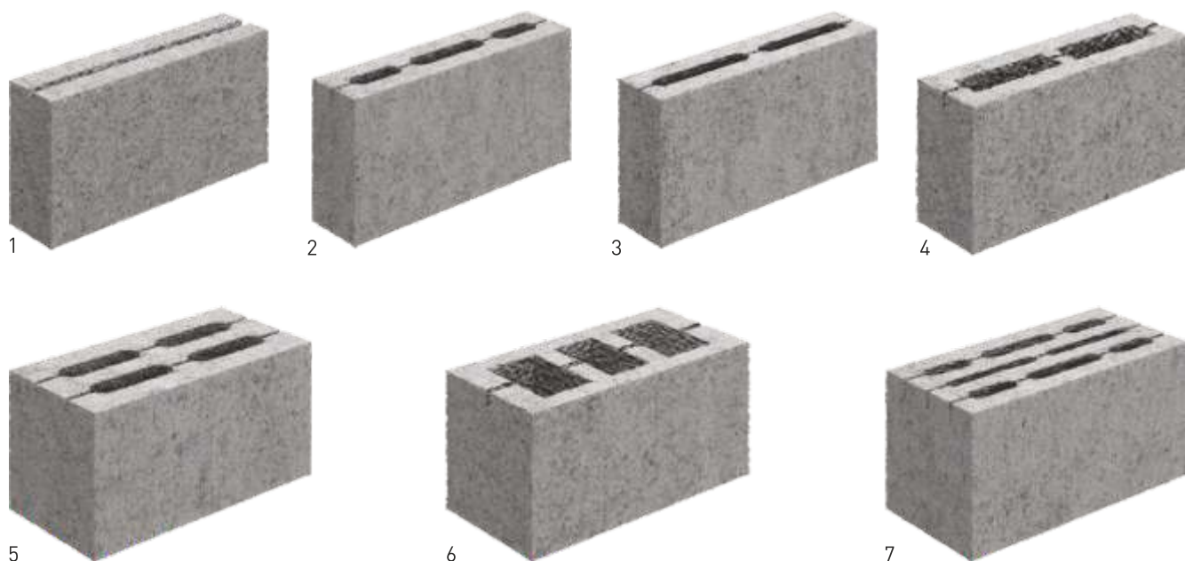
1 390X90X188 2 390X90X188
