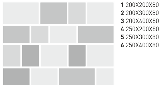
БЕНИЛЮКС МУЛЬТИФОРМАТ 6 1200X900X80
